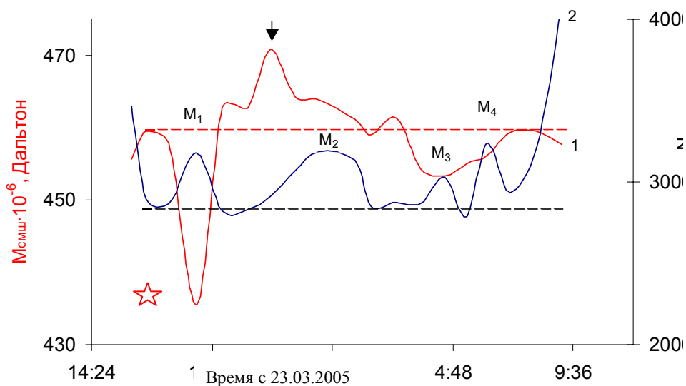
Рис. 7. Характер изменения средней молекулярной массы (1) кластеров (ансамбль до 4 млрд. Дальтон) и числа их видов (2) в водном растворе поваренной соли (3.5 вес. % NaCl). Пунктирные линии – базовые линии средних значений.
